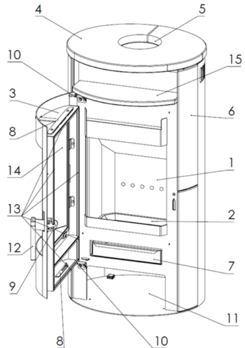
Abbildung 1 – Aufbau des Geräts
