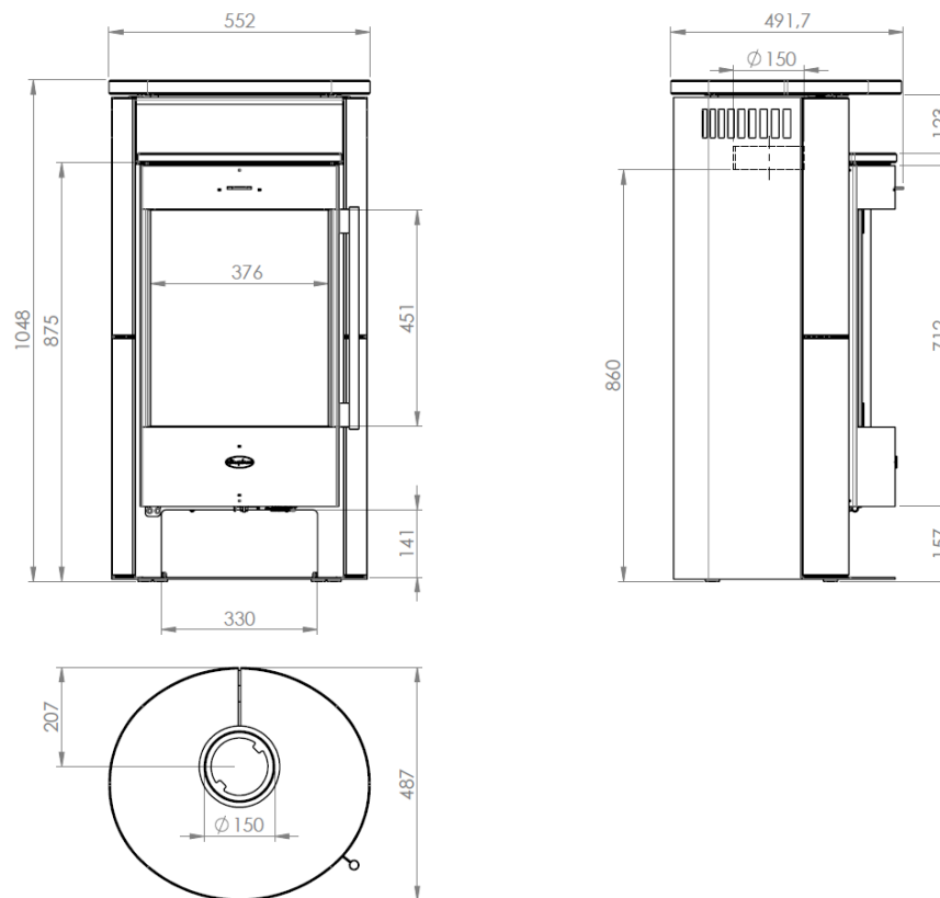
Abbildung 6 - Hauptmaße
