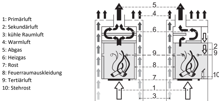
Abbildung 12 – Fire-Plus System, schematische Darstellung
