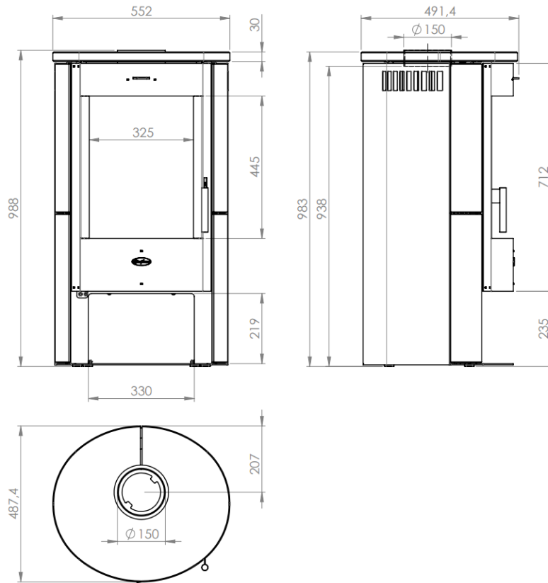
Abbildung 3 – Hauptmaße
