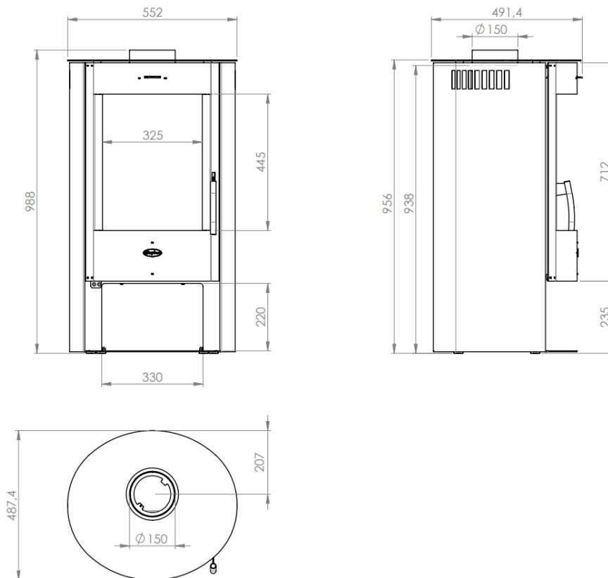
Abbildung 4 – Hauptmaße
