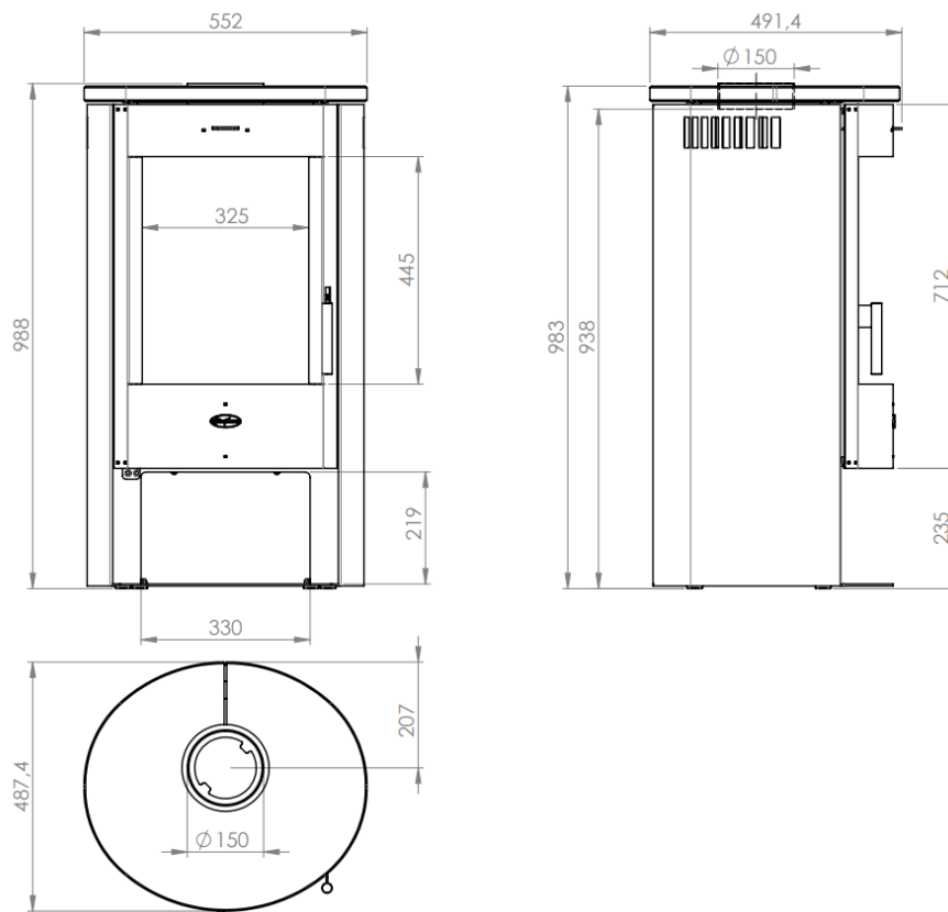
Abbildung 10 - Hauptmaße
