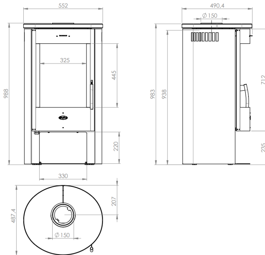
Abbildung 5 - Hauptmaße
