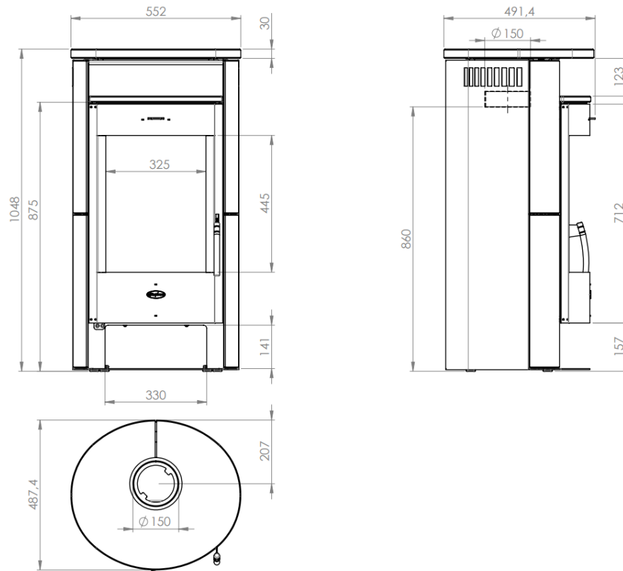
Abbildung 7 – Hauptmaße
