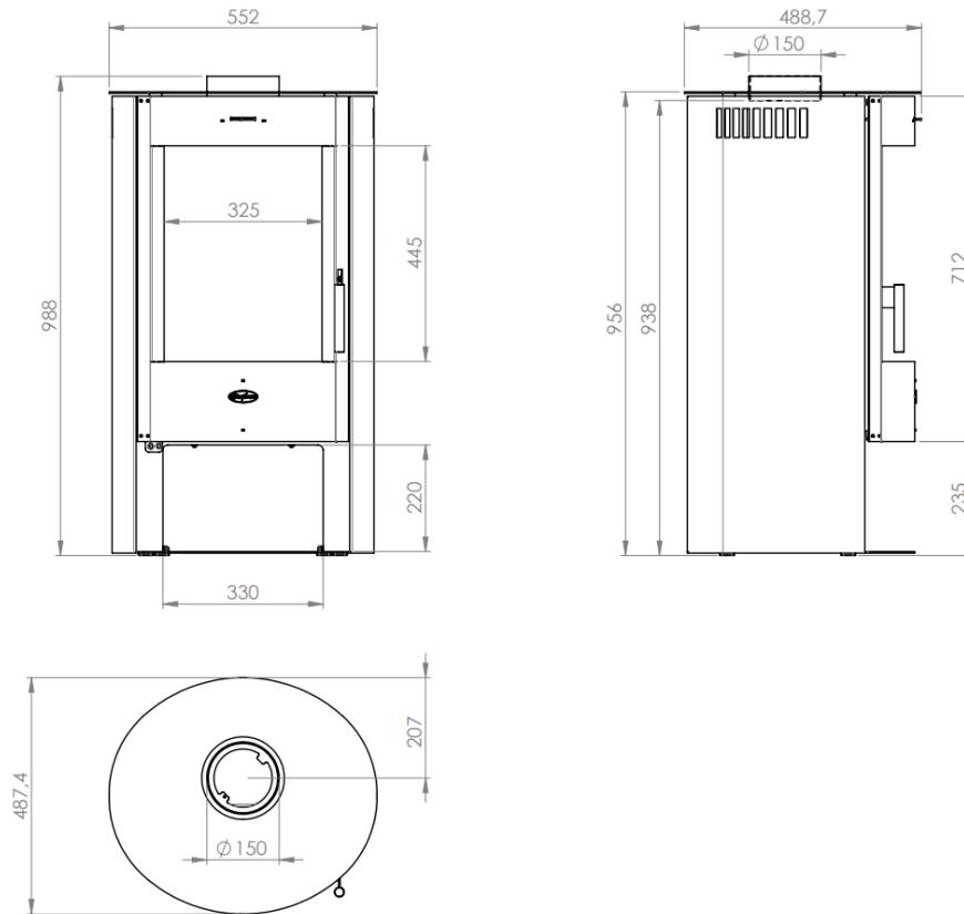
Abbildung 11 - Hauptmaße
