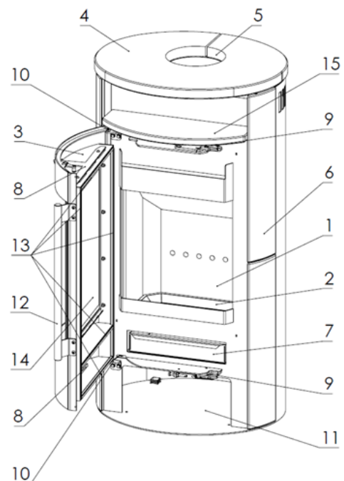
Abbildung 2 - Aufbau des Geräts /R5688 & R5693/
