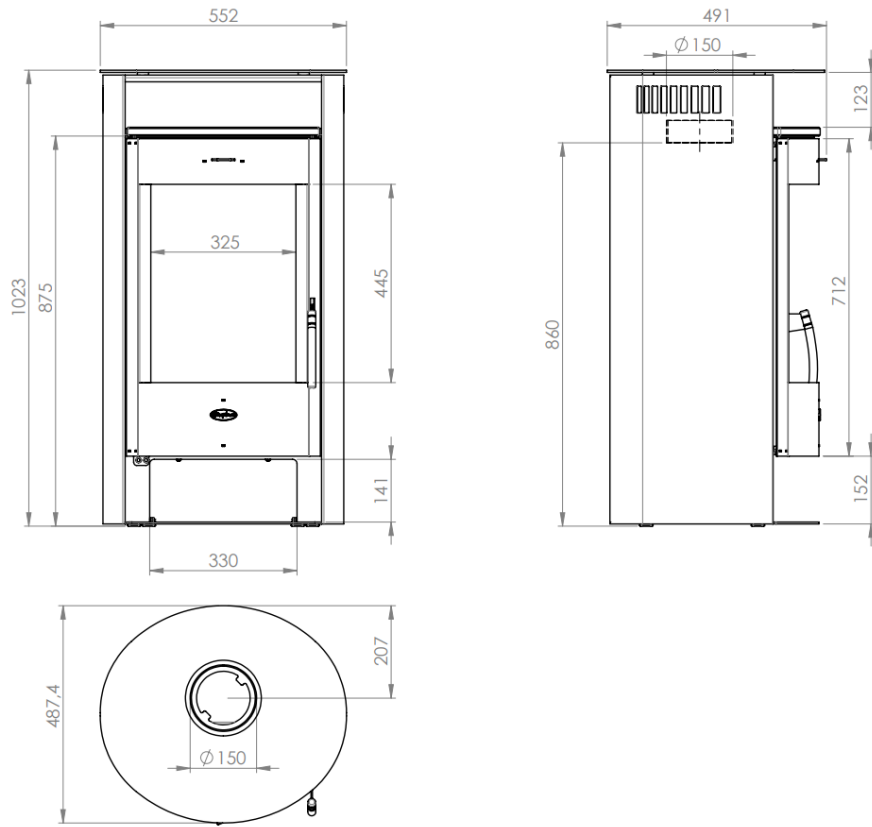
Abbildung 9 - Hauptmaße
