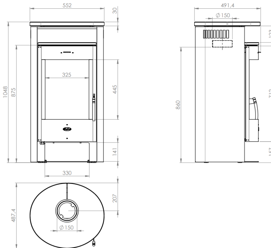
Abbildung 8 - Hauptmaße
