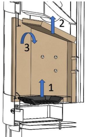
Abbildung 12 – Zugang zum Rauchraum
