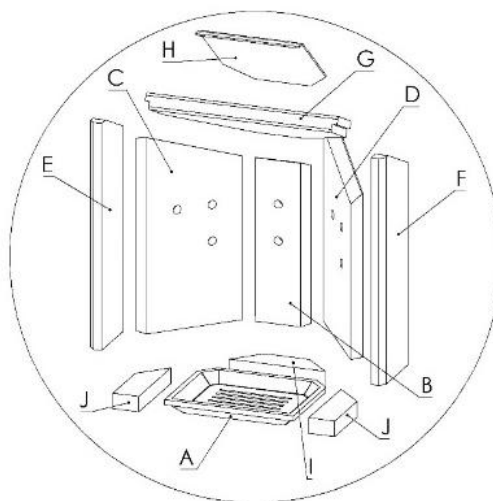
Abbildung 11 – Feuerraumauskleidung mit Rost
