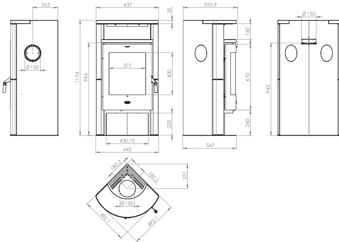
Abbildung 2 - Hauptmaße
