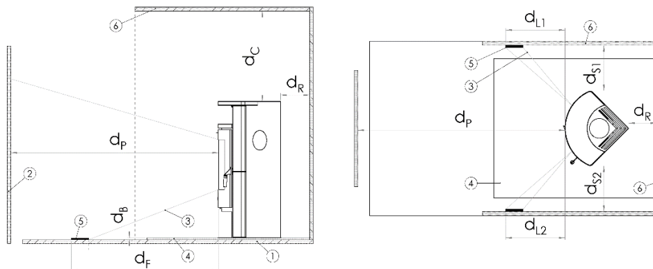
Abbildung 7 - Schematische Darstellung der Mindestabstände (siehe Tabelle 2)
