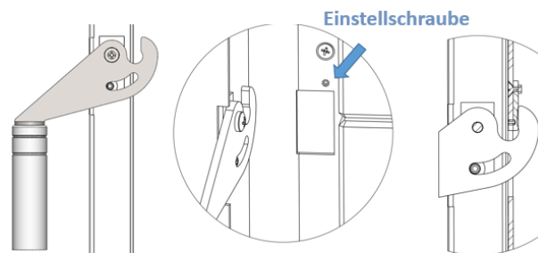
Abbildung 13 - Verriegelung
