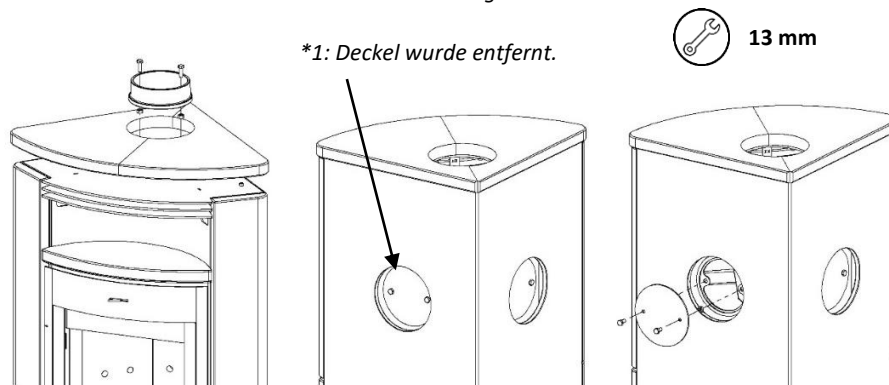
Abbildung 5 - Abgasstutzen und Abdeckung demontieren
