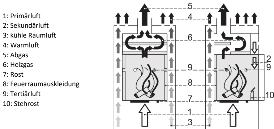
Abbildung 4 – Fire-Plus System, schematische Darstellung
