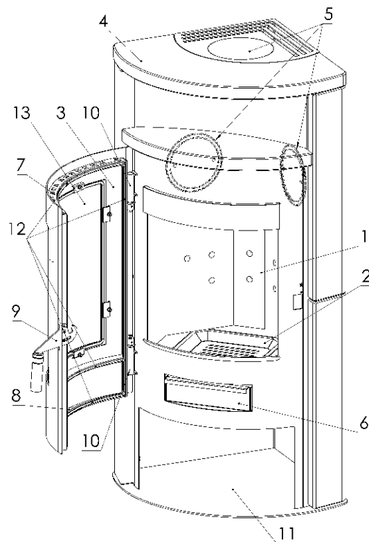
Abbildung 1 – Aufbau des Geräts
