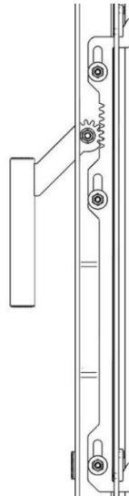
Abbildung 16 - Merfachverriegelung
