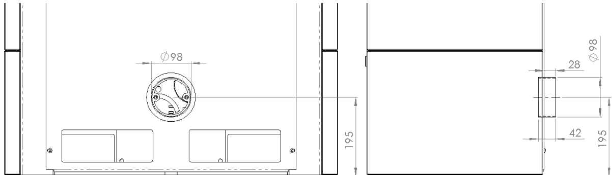
Abbildung 7- Verbrennungsluftanschluss
