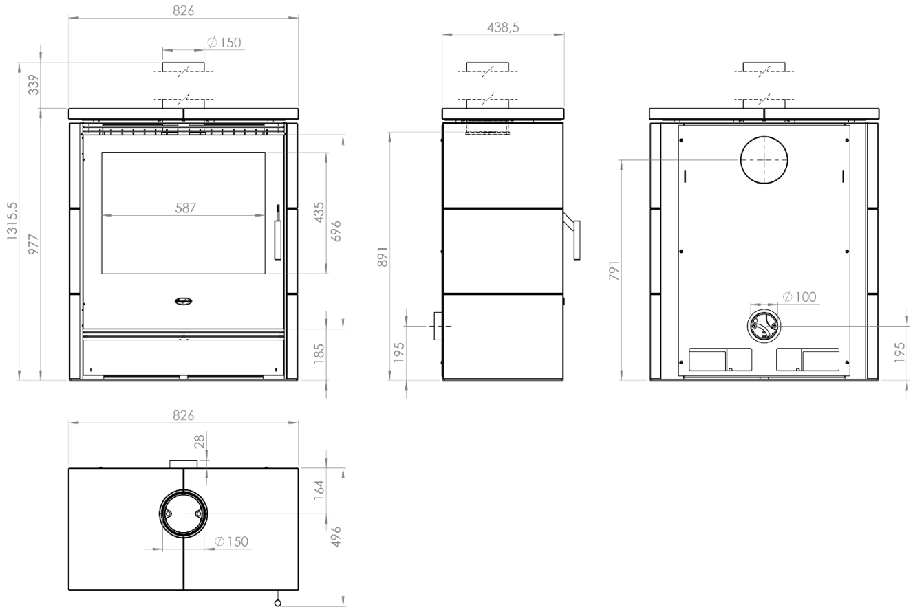
Abbildung 2 – Hauptmaße
