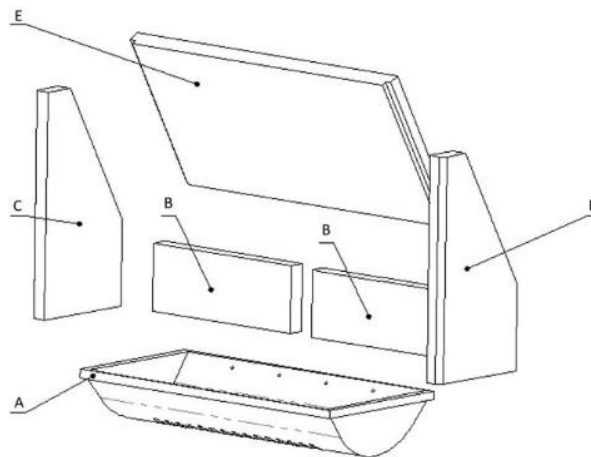
Abbildung 14 – Feuerraumauskleidung mit Rost
