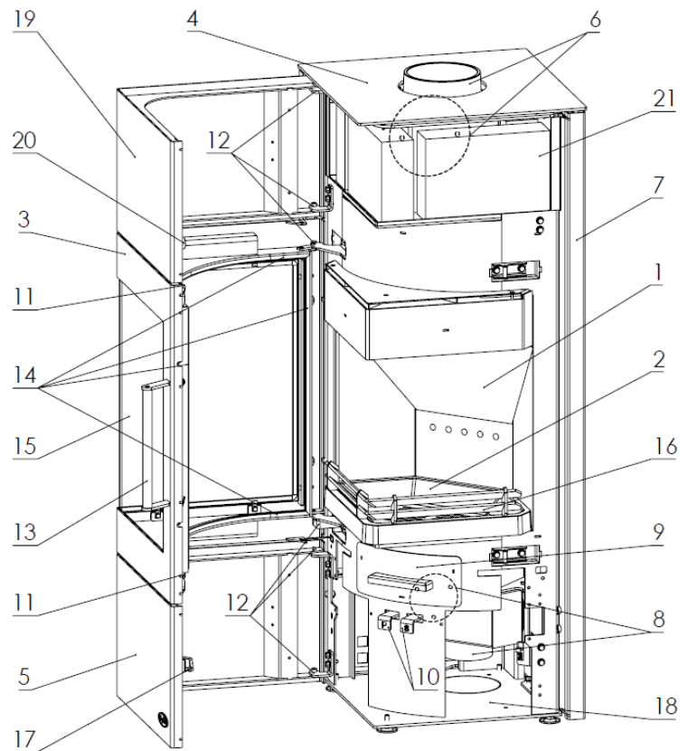
Abbildung 1 – Aufbau des Geräts K6490
