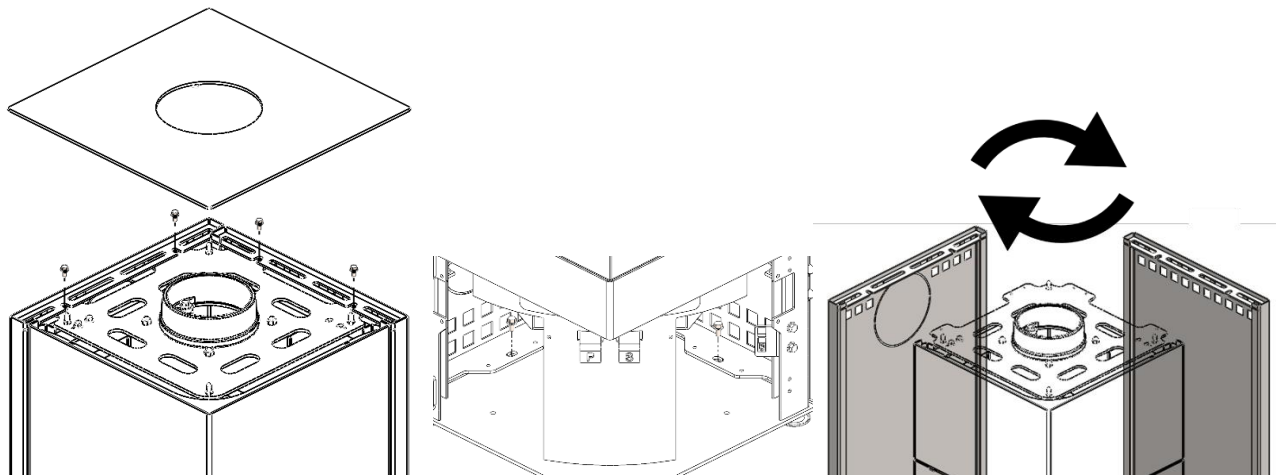
Abbildung 9 – Austausch der Seitenverkleidungen
