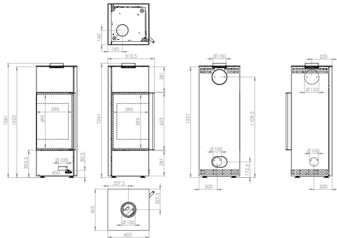
Abbildung 4 - Hauptmaße
