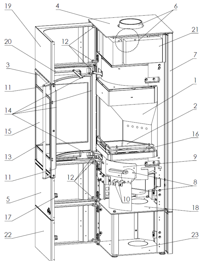
Abbildung 2 – Aufbau des Geräts K6495
