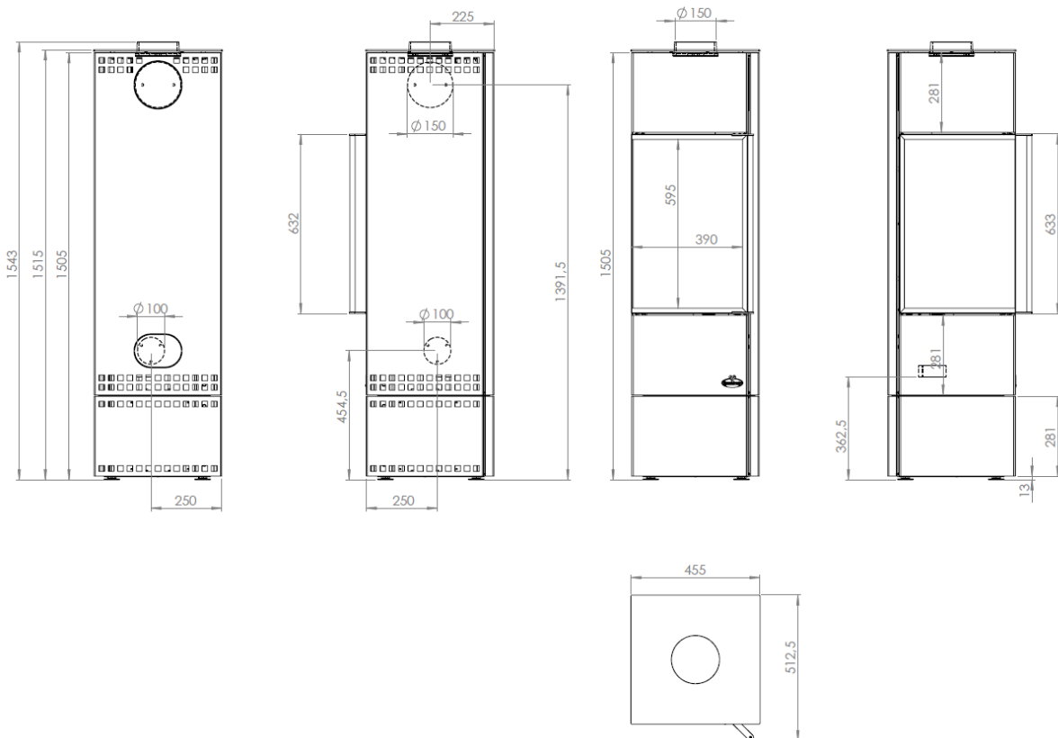
Abbildung 5 - Hauptmaße
