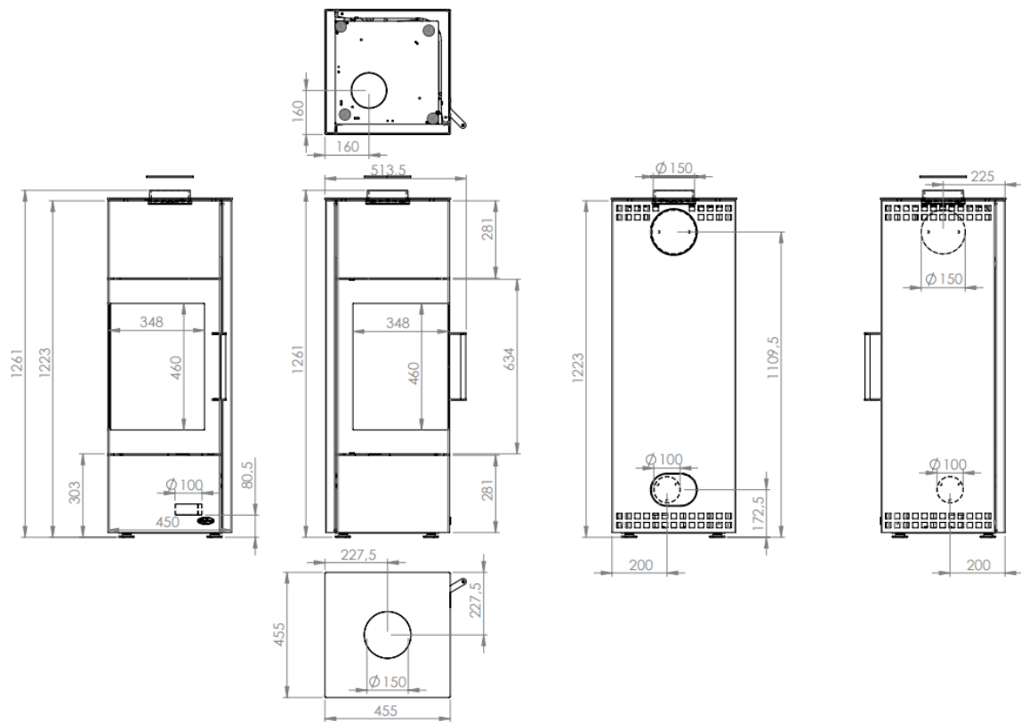
Abbildung 3 - Hauptmaße
