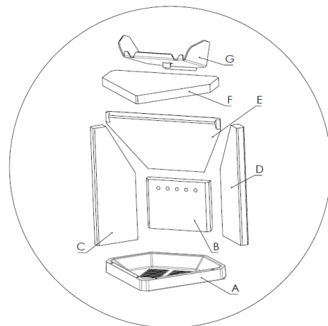
Abbildung 16 – Feuerraumauskleidung mit Rost
