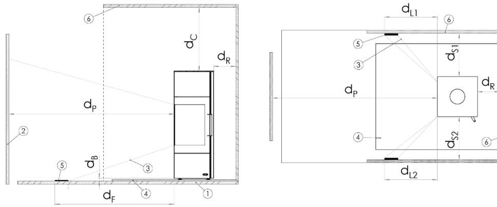
Abbildung 12 - Schematische Darstellung der Mindestabstände (siehe Tabelle 2)
