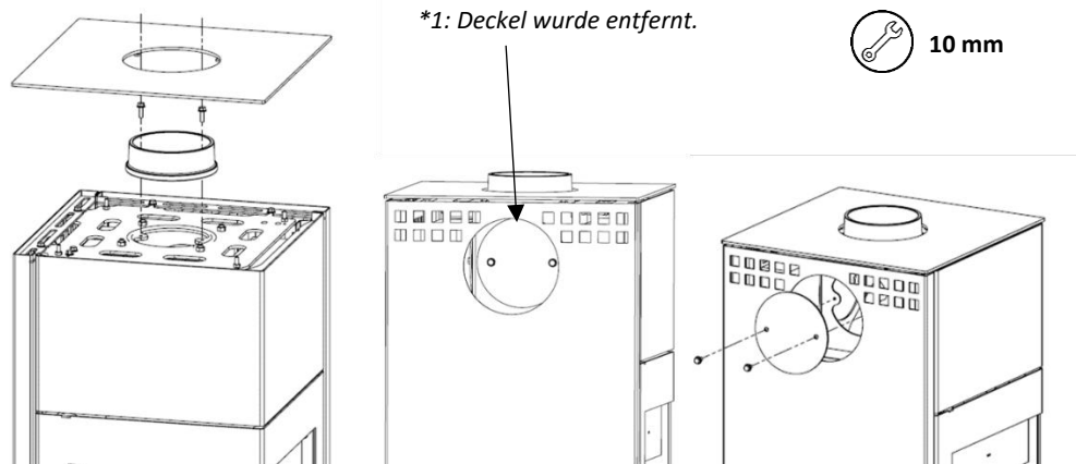
Abbildung 7 - Abgasstutzen und Abdeckung demontieren
