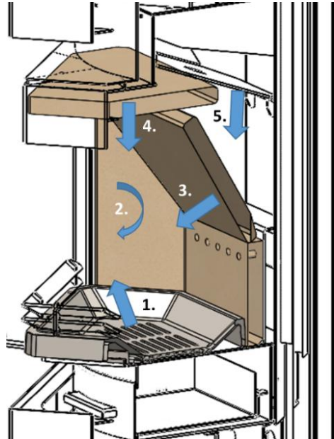
Abbildung 17 – Zugang zum Rauchraum
