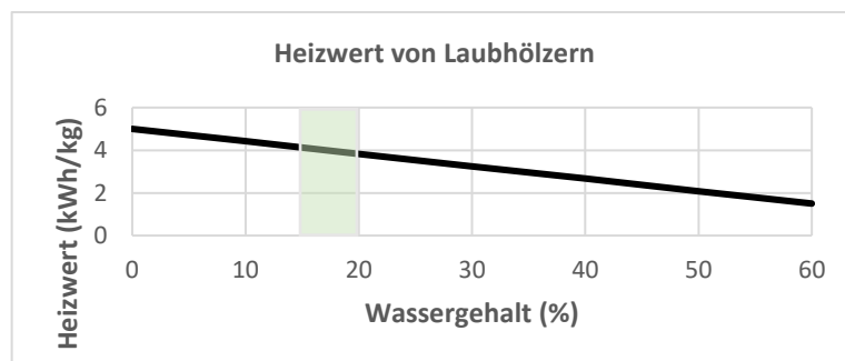
Abbildung 13 - Heizwertänderung in Abhängigkeit vom Wassergehalt
