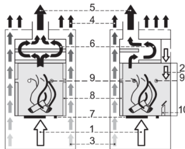
Abbildung 6 – Fire-Plus System, schematische Darstellung
