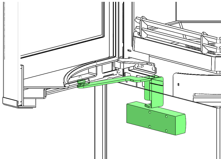
Abbildung 19 - Hydraulischer Türverschluss
