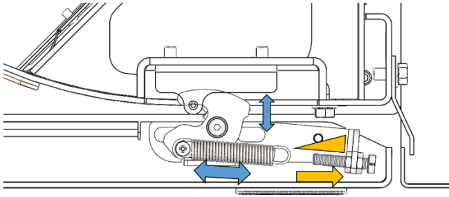
Abbildung 18 – Schnappverschluss
