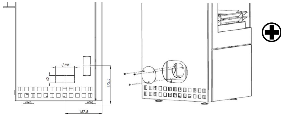
Abbildung 8- Verbrennungsluftanschluss
