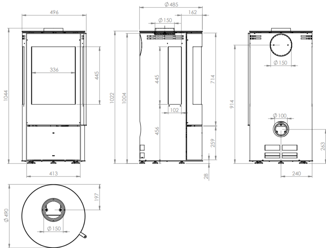
Abbildung 2 - Hauptmaße
