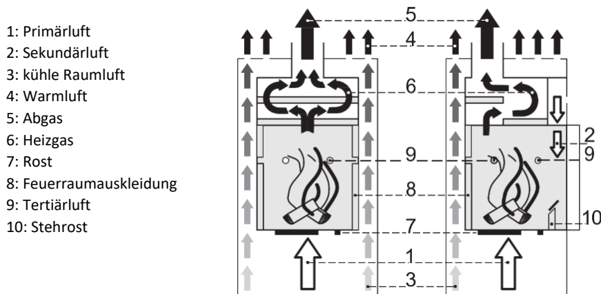
Abbildung 5 – Fire-Plus System, schematische Darstellung
