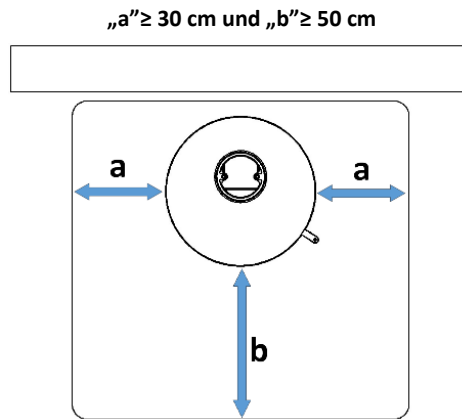
Abbildung 8 - Bodenplatte
