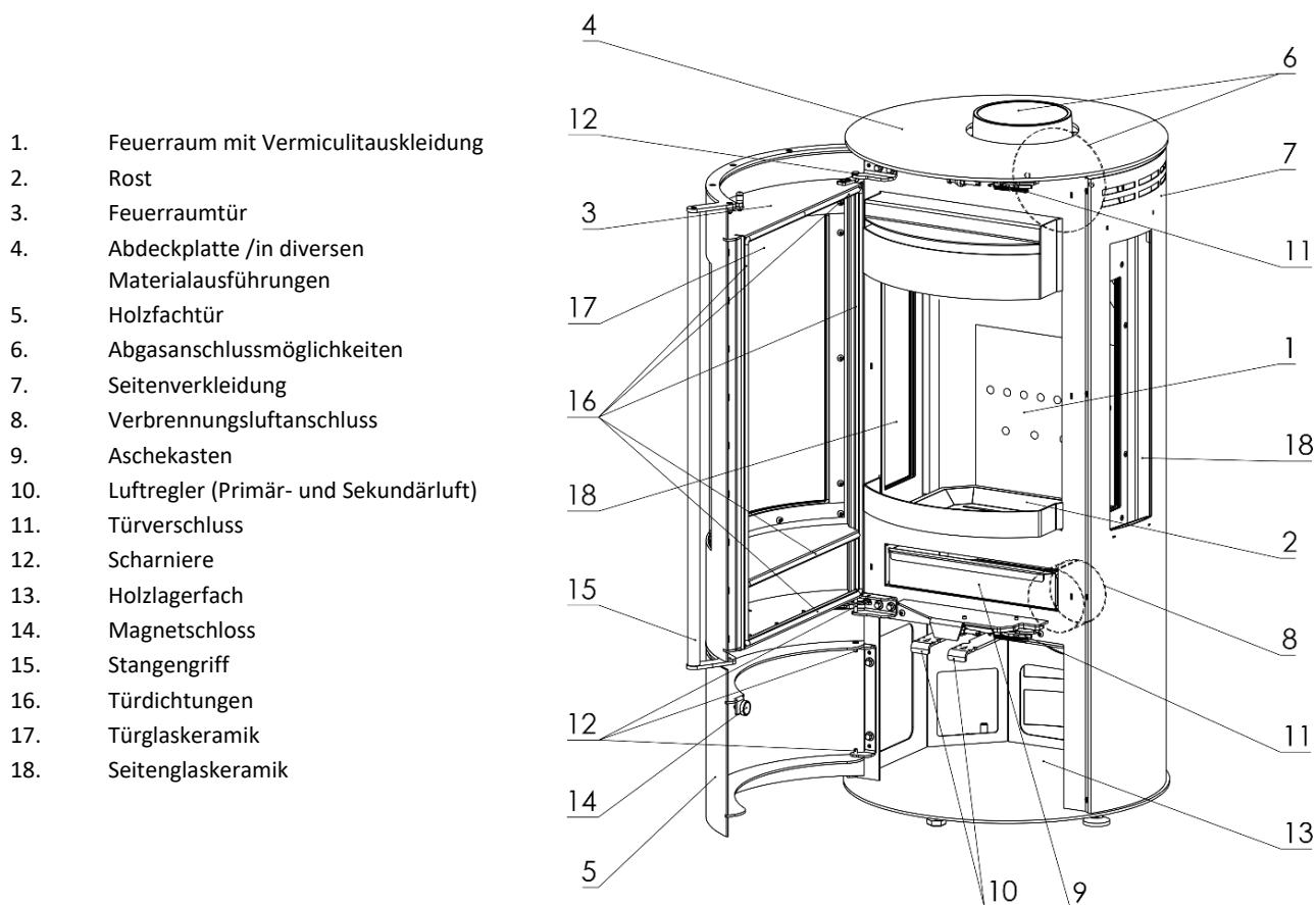
Abbildung 1 – Aufbau des Geräts
