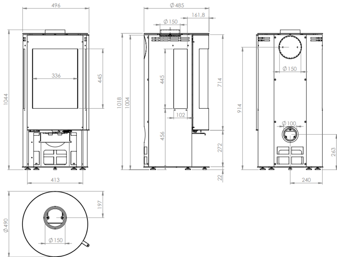
Abbildung 4 - Hauptmaße
