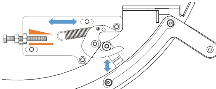
Abbildung 15 - Schnappverschluss
