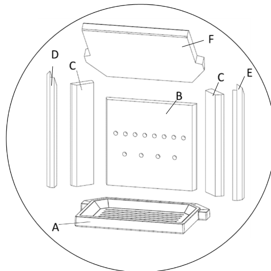
Abbildung 13 – Feuerraumauskleidung mit Rost
