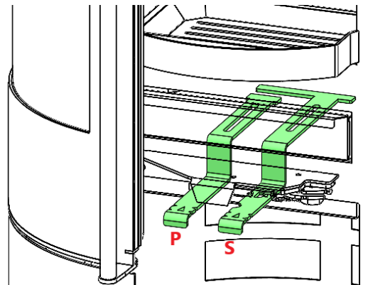
Abbildung 12 - P: Primärluftregler, S: Sekundärluftregler
