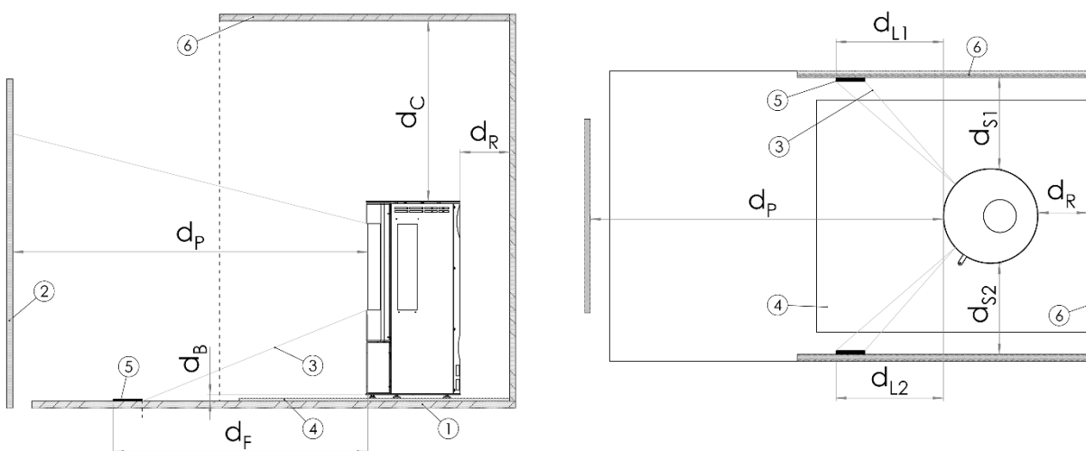
Abbildung 9 - Schematische Darstellung der Mindestabstände (siehe Tabelle 2)
