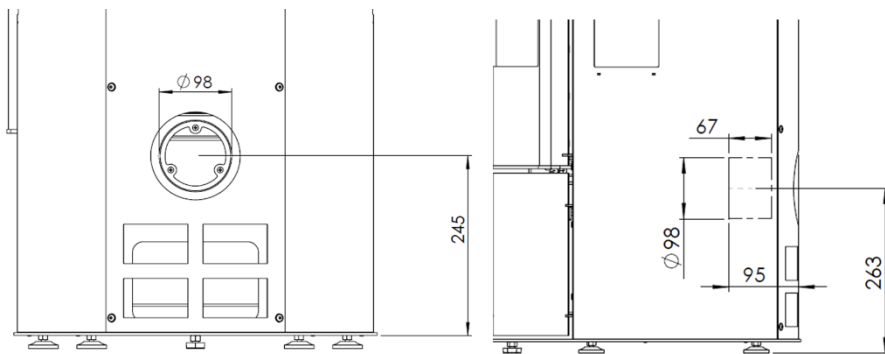
Abbildung 7- Verbrennungsluftanschluss
