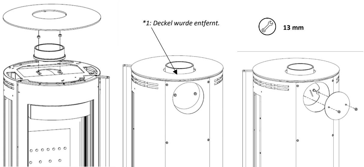
Abbildung 6 - Abgasstutzen und Abdeckung demontieren
