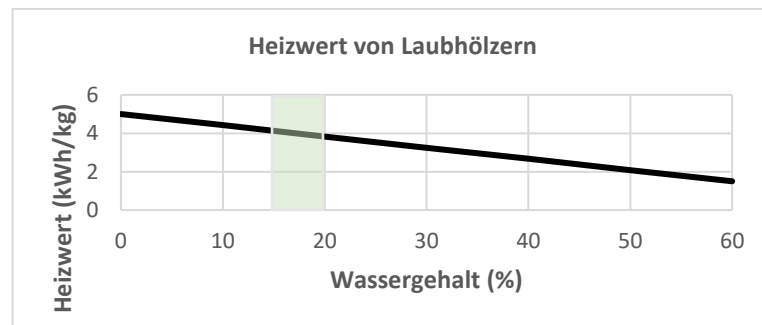
Abbildung 15 - Heizwertänderung in Abhängigkeit vom Wassergehalt
