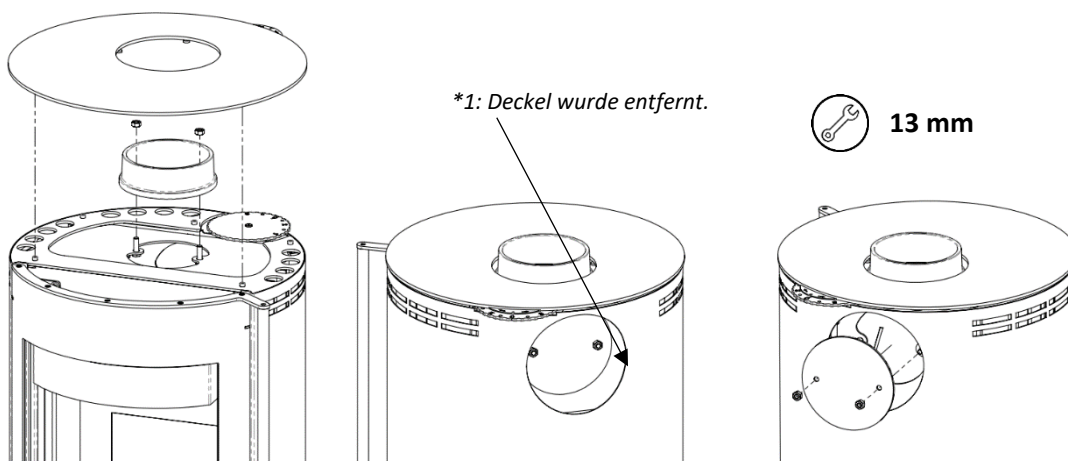
Abbildung 10 - Abgasstutzen und Abdeckung demontieren
