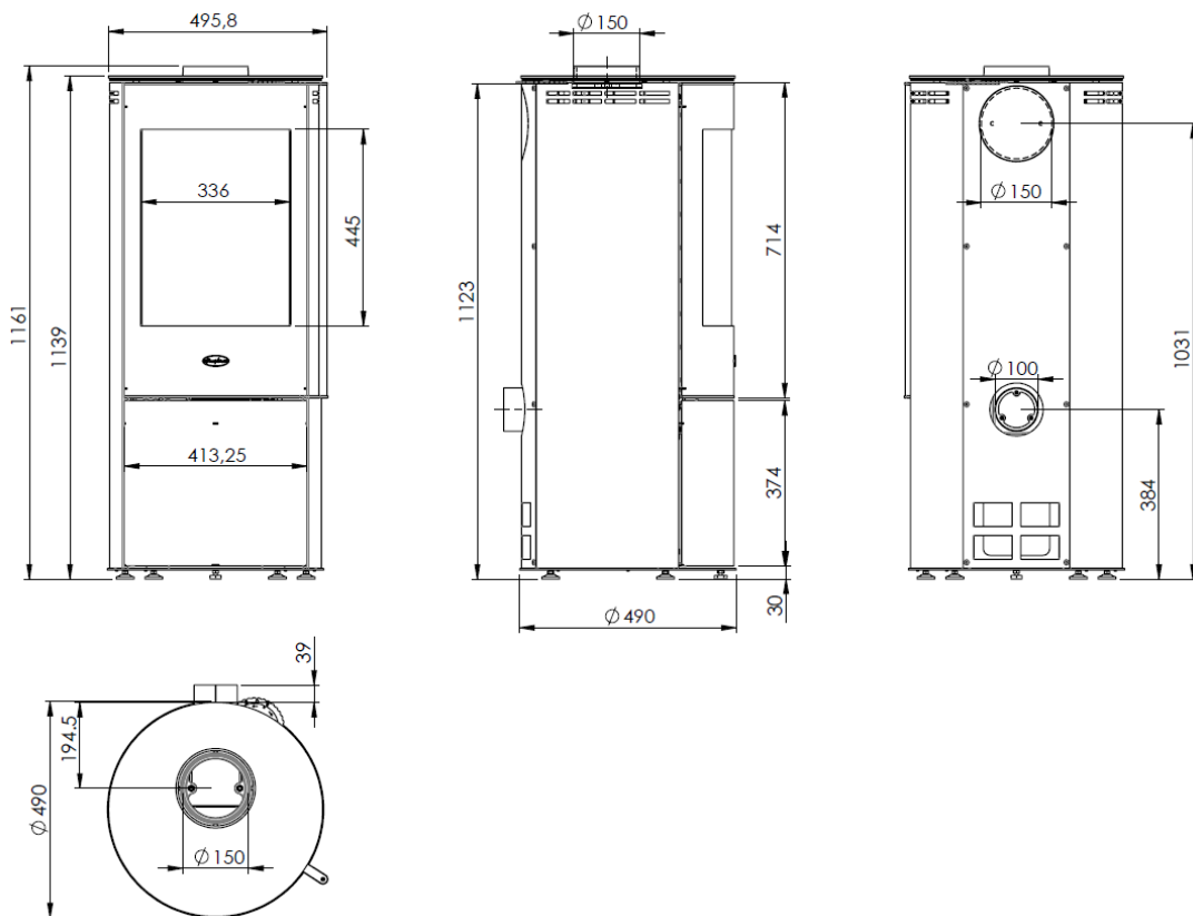
Abbildung 3 - Hauptmaße
