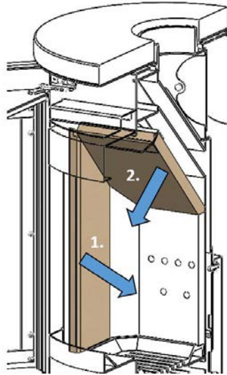
Abbildung 20 – Zugang zum Rauchraum
