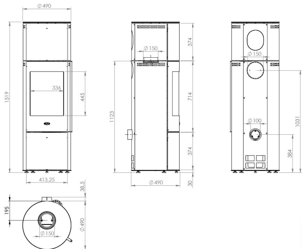
Abbildung 7 - Hauptmaße
