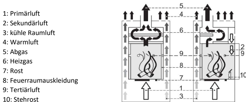
Abbildung 9 – Fire-Plus System, schematische Darstellung
