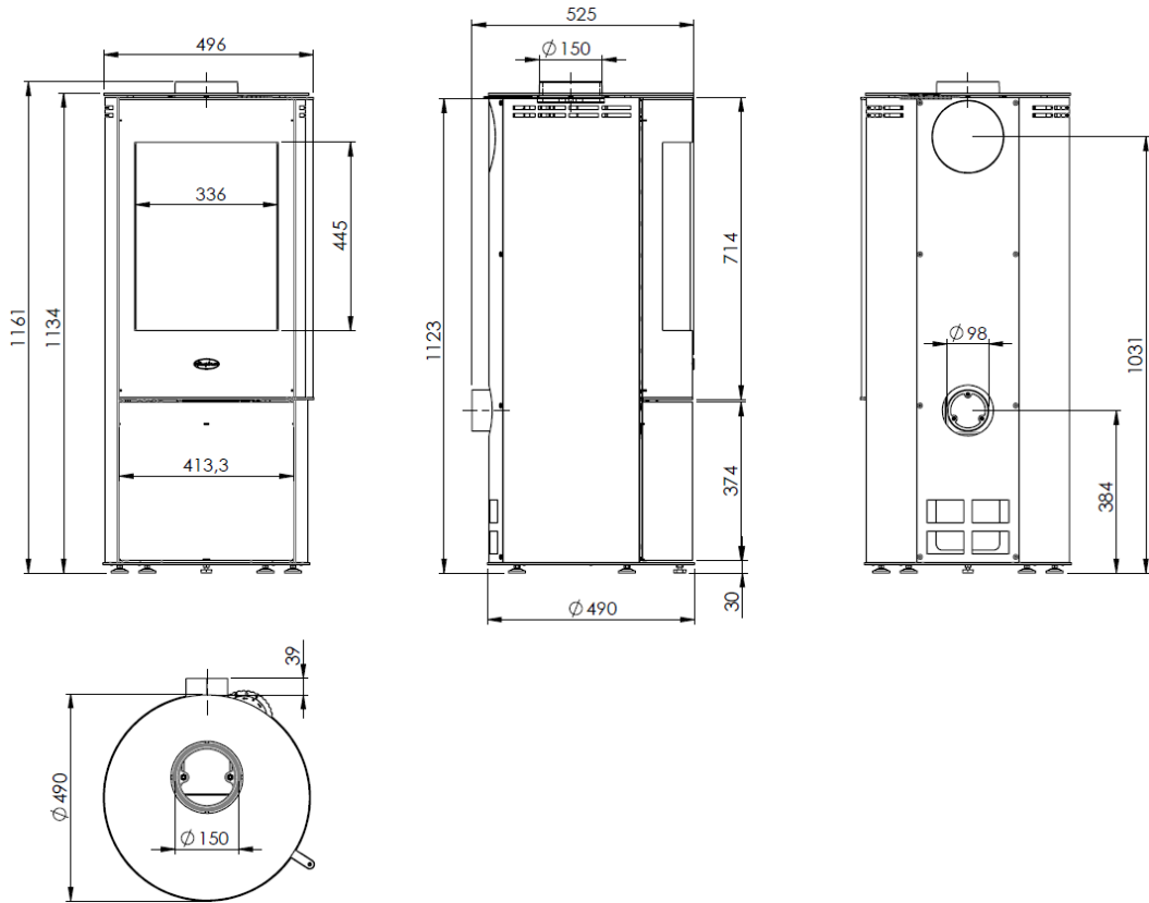
Abbildung 2 - Hauptmaße
