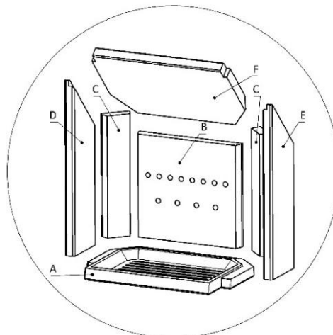
Abbildung 19 – Feuerraumauskleidung mit Rost
