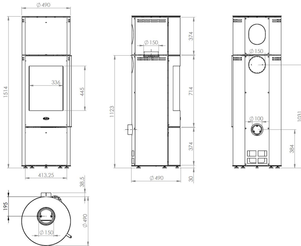
Abbildung 6 - Hauptmaße
