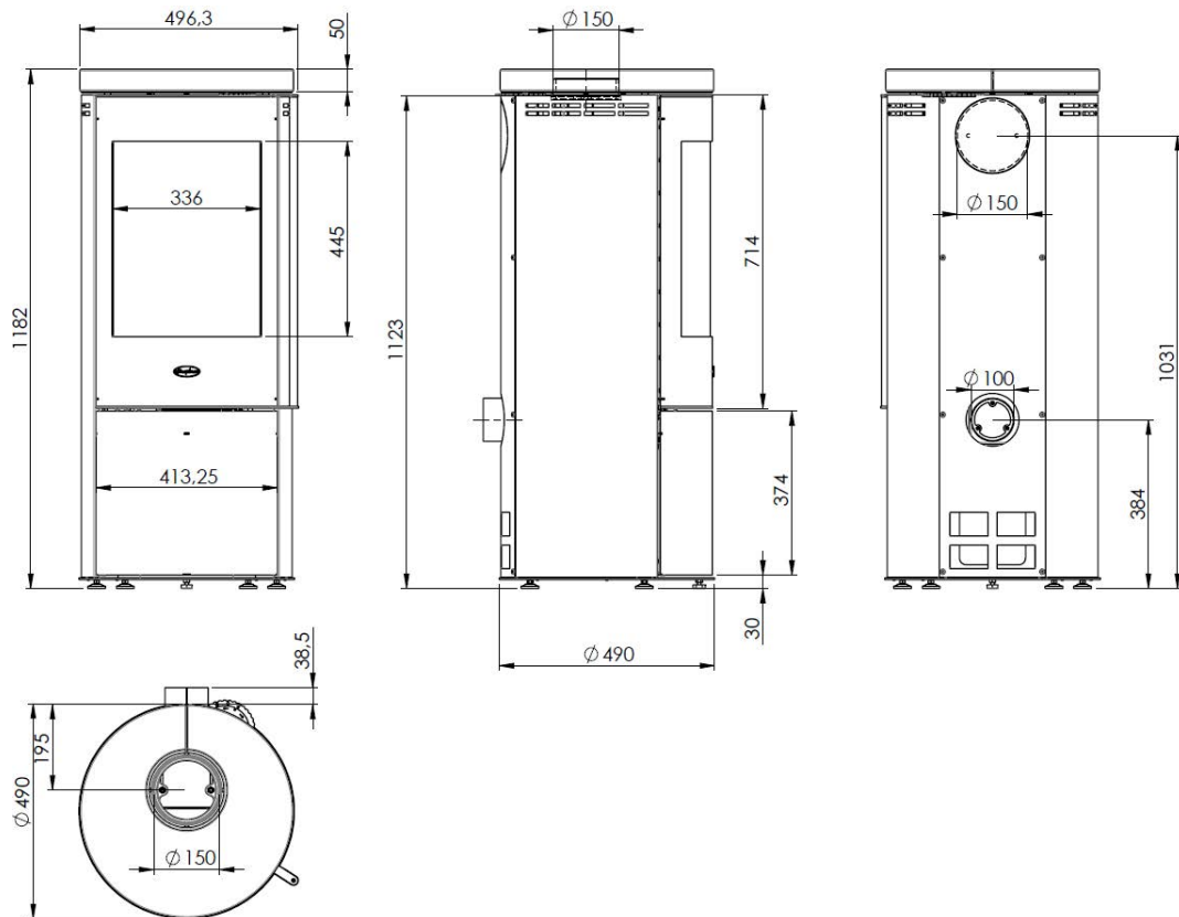
Abbildung 5 – Hauptmaße
