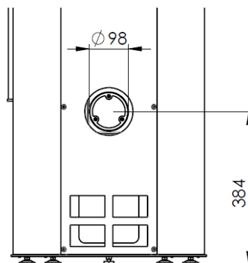
Abbildung 11- Verbrennungsluftanschluss
