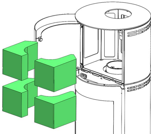
Abbildung 12 – Wärmespeichersteine
