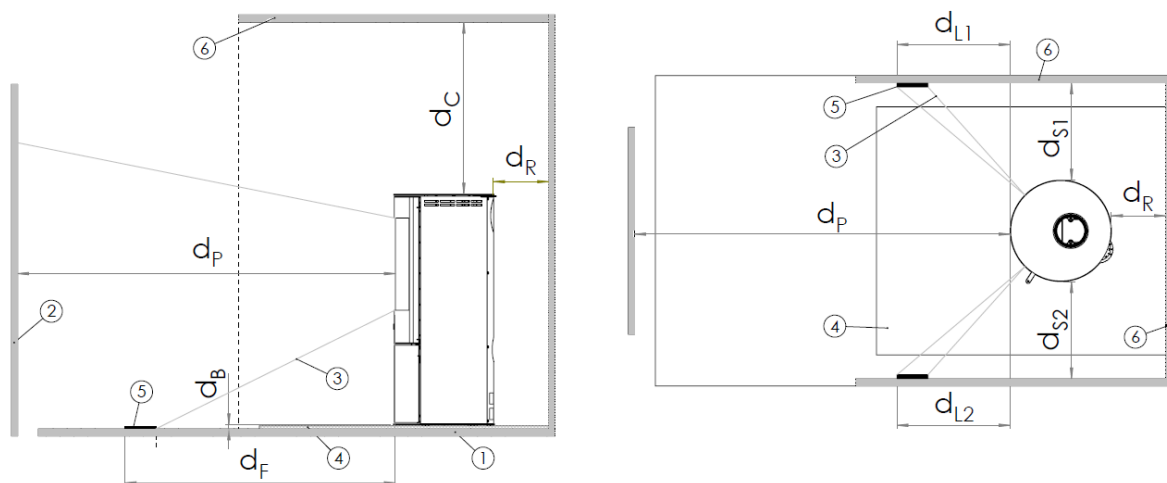
Abbildung 14 - Schematische Darstellung der Mindestabstände (siehe Tabelle 2)
