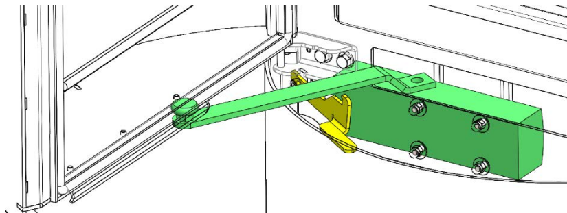
Abbildung 21 – Hydraulischer Türverschluss
