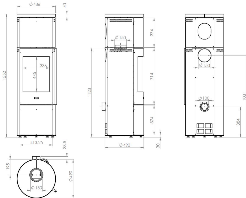
Abbildung 8 - Hauptmaße
