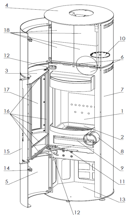
Abbildung 1 – Aufbau des Geräts
