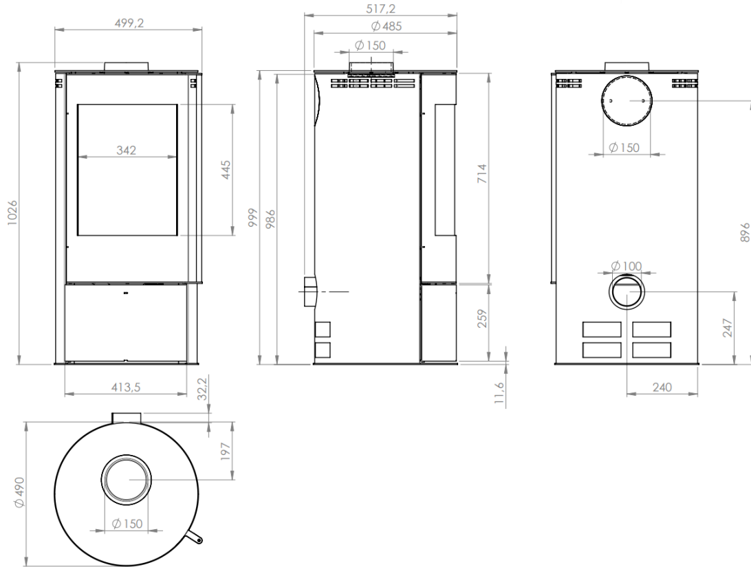
Abbildung 2 - Hauptmaße
