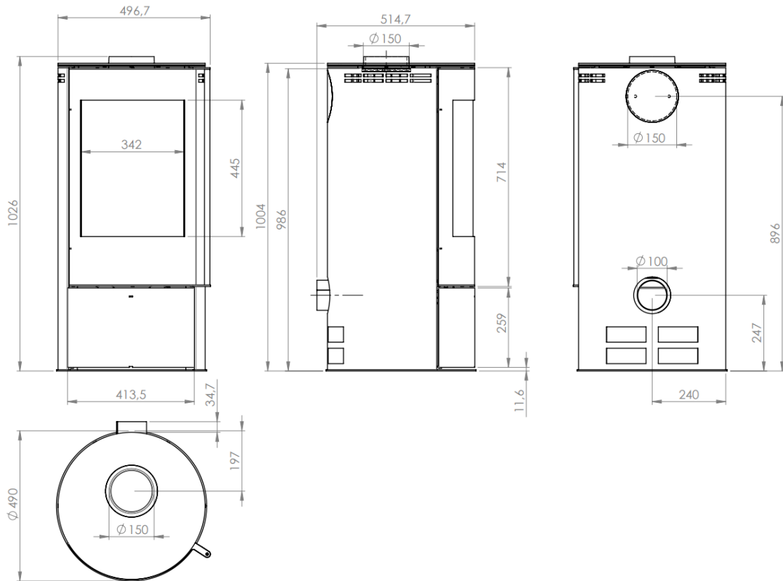
Abbildung 3 - Hauptmaße
