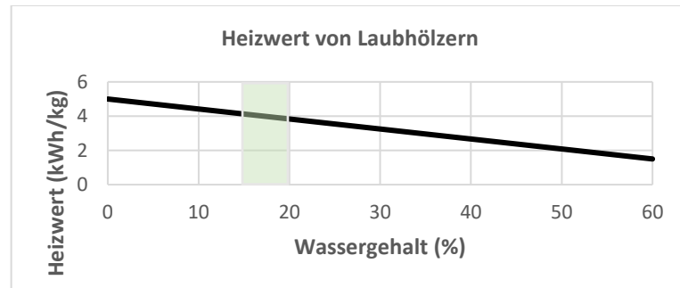
Abbildung 11 - Heizwertänderung in Abhängigkeit vom Wassergehalt
