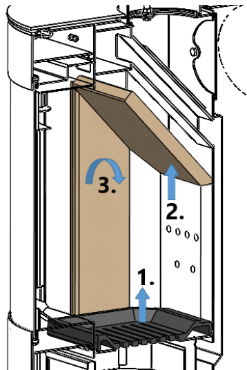
Abbildung 15 – Zugang zum Rauchraum
