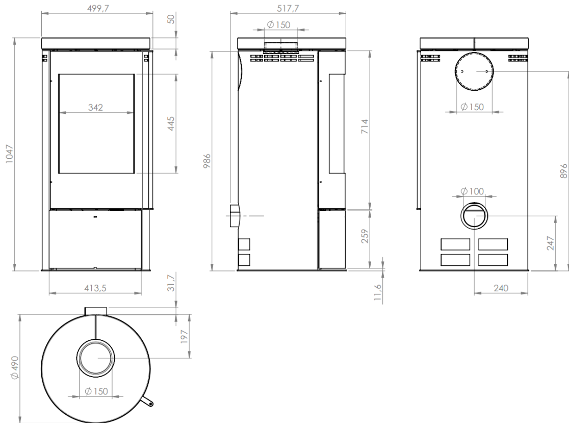
Abbildung 5 - Hauptmaße
