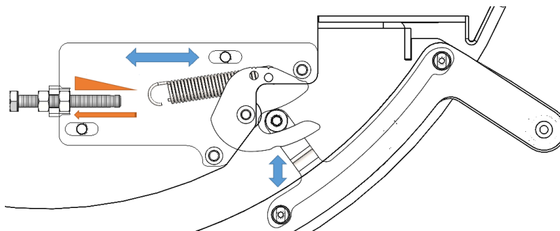
Abbildung 16 - Schnappverschluss
