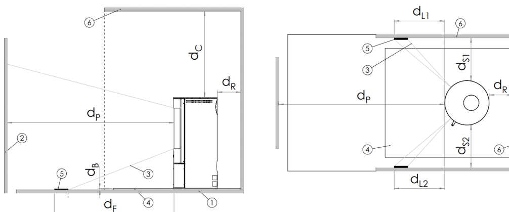
Abbildung 10 - Schematische Darstellung der Mindestabstände (siehe Tabelle 2)
