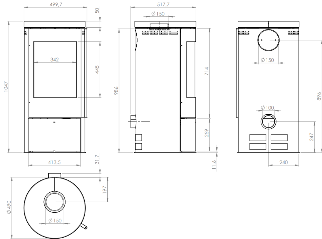
Abbildung 4 - Hauptmaße
