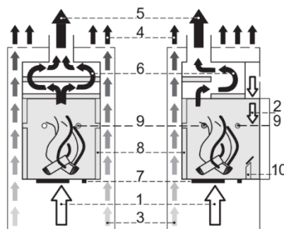
Abbildung 6 – Fire-Plus System, schematische Darstellung
