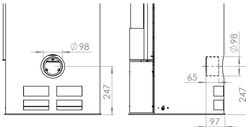
Abbildung 8- Verbrennungsluftanschluss
