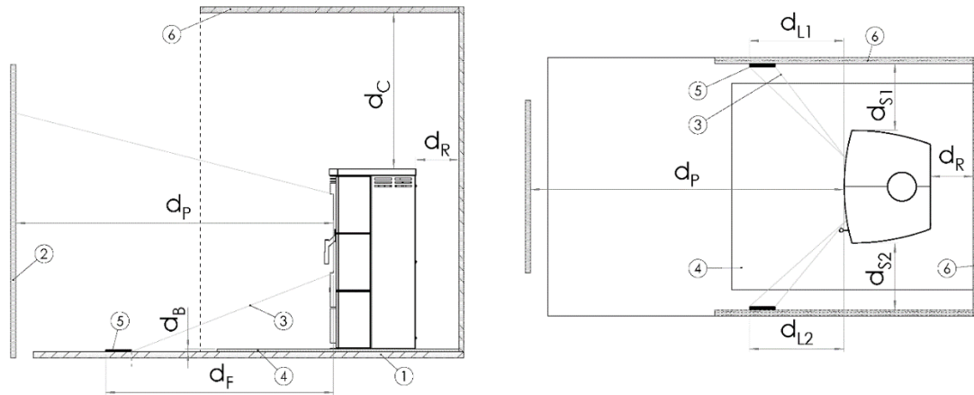
Abbildung 7 - Schematische Darstellung der Mindestabstände (siehe Tabelle 2)
