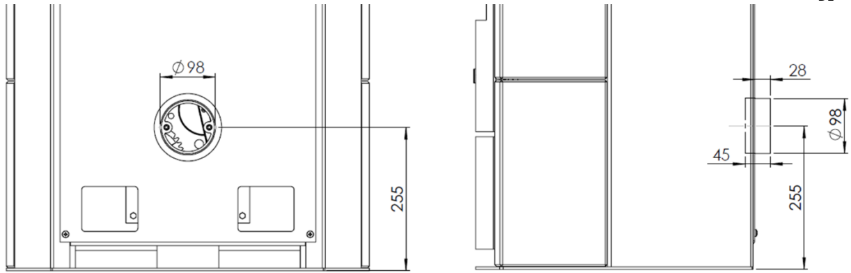
Abbildung 5 - Verbrennungsluftanschluss
