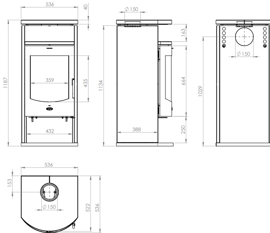
Abbildung 3 - Hauptmaße
