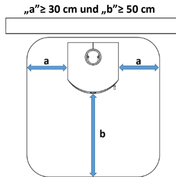
Abbildung 6 - Bodenplatte
