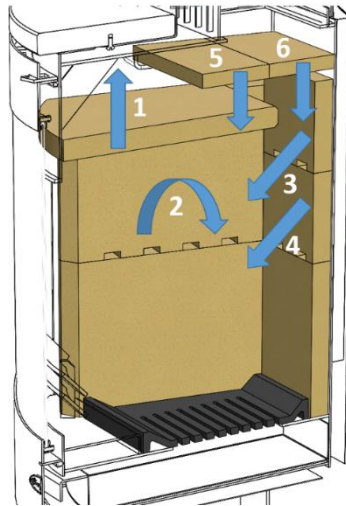
Abbildung 12 – Zugang zum Rauchraum
