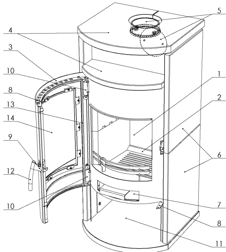
Abbildung 1 – Aufbau des Geräts
