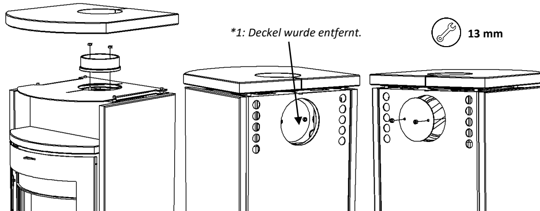
Abbildung 5 - Abgasstutzen und Abdeckung demontieren
