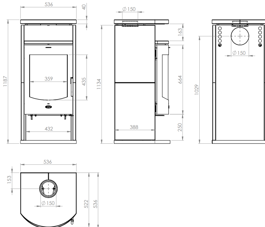
Abbildung 2 - Hauptmaße
