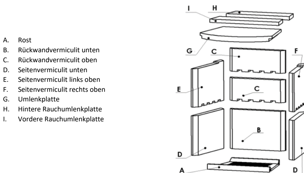
Abbildung 11 – Feuerraumauskleidung mit Rost
