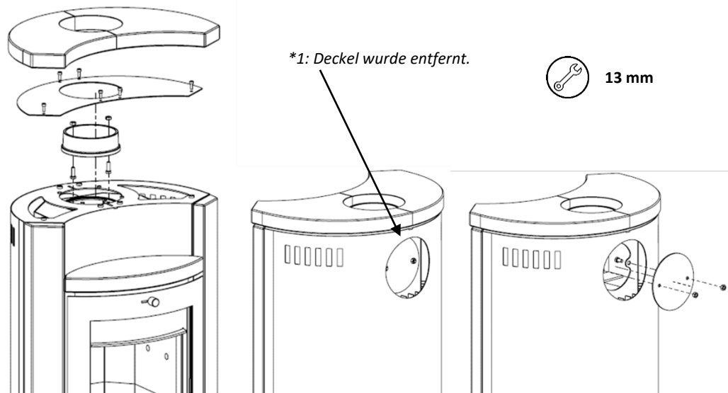
Abbildung 4 - Abgasstutzen und Abdeckung demontieren
