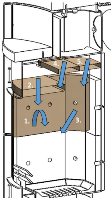
Abbildung 11 – Zugang zum Rauchraum
