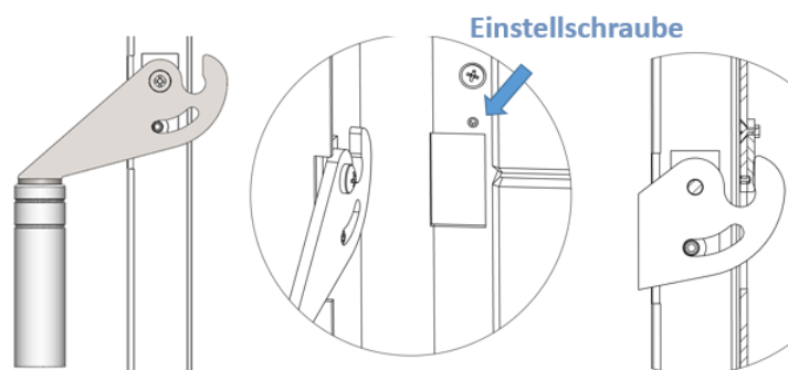
Abbildung 12 - Verriegelung
