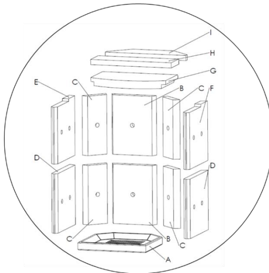
Abbildung 10 – Feuerraumauskleidung mit Rost
