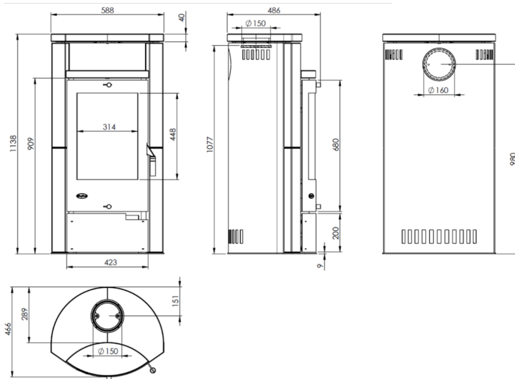
Abbildung 2 - Hauptmaße
