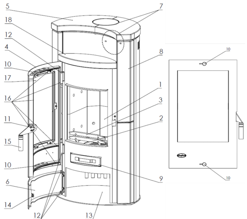
Abbildung 1 – Aufbau des Geräts
