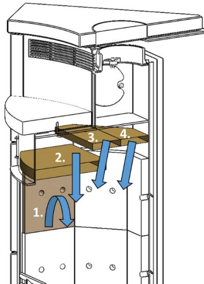
Abbildung 12 – Zugang zum Rauchraum
