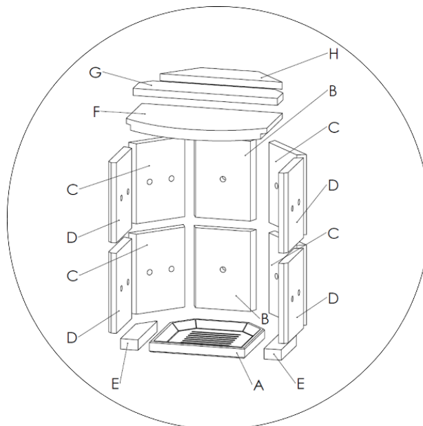
Abbildung 11 – Feuerraumauskleidung mit Rost
