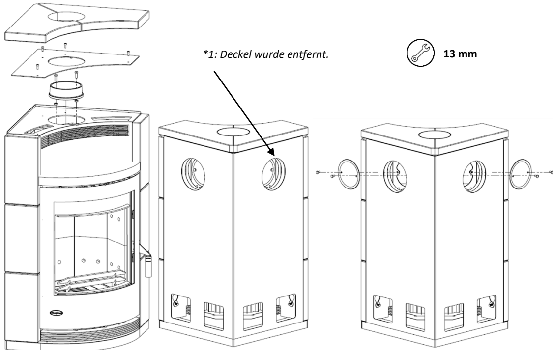
Abbildung 5 - Abgasstutzen und Abdeckung demontieren
