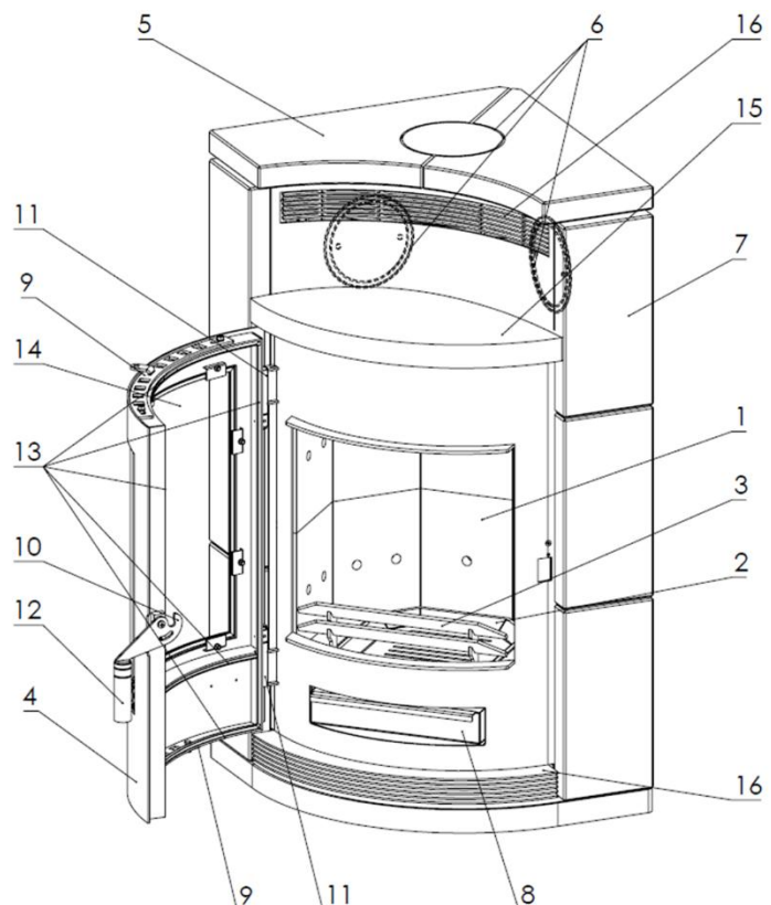
Abbildung 1 – Aufbau des Geräts
