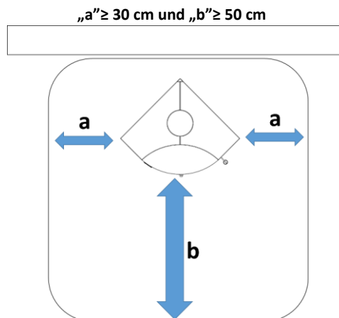
Abbildung 6 - Bodenplatte
