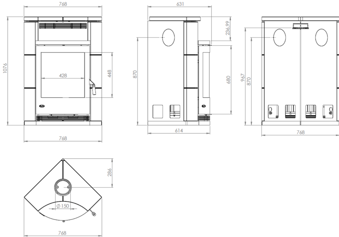
Abbildung 2 - Hauptmaße
