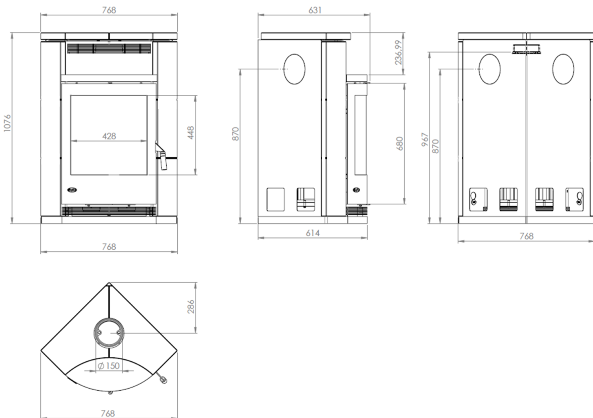
Abbildung 3 - Hauptmaße
