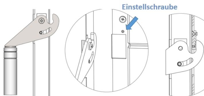
Abbildung 13 - Verriegelung
